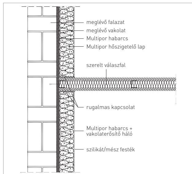
Szerelt válaszfal – vízszintes (a)
