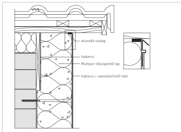
Ereszcsatlakozás 1.
