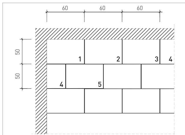
Beépítési sorrend
