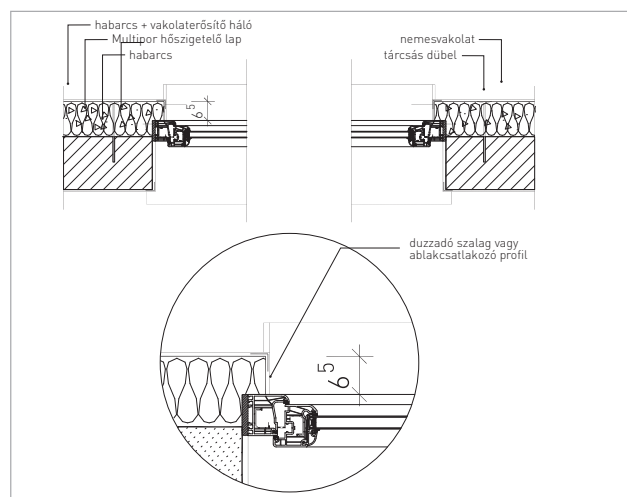
Nyílászáró – vízszintes
