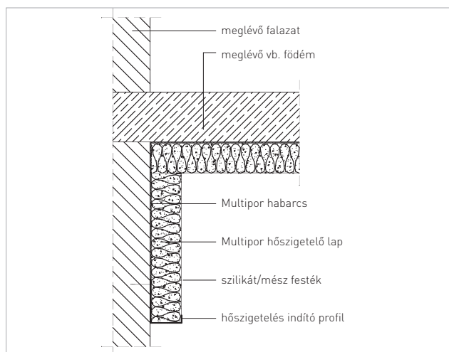
Födém – fal csatlakozás 2.
