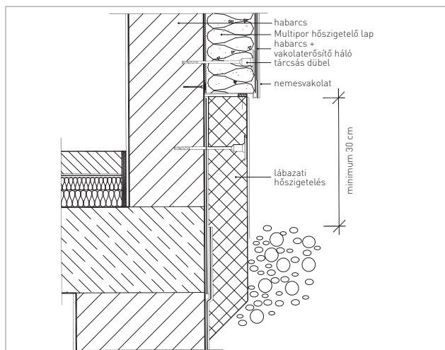
Lábazatkialakítás
