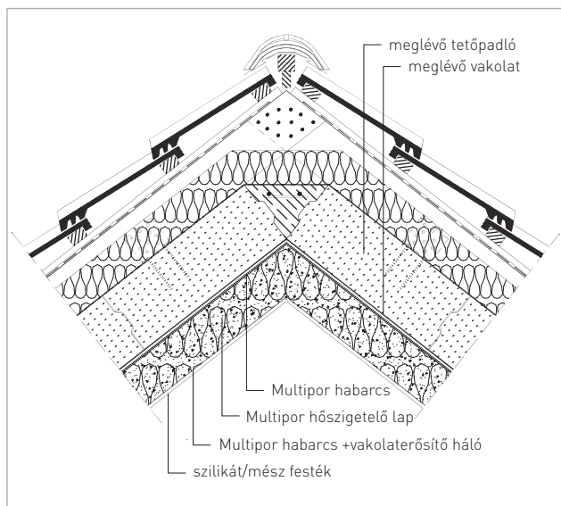
Tetőtér pallófödém 3.
