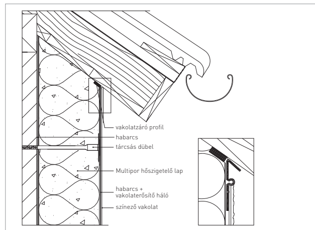
Ereszcsatlakozás 2.
