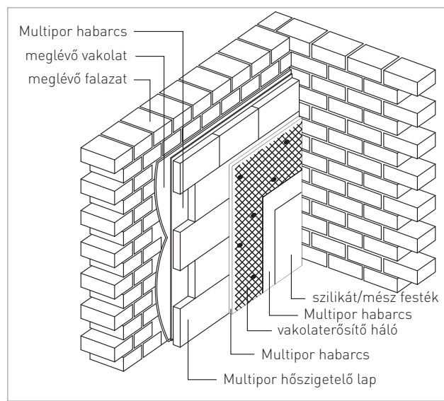
Rétegrend
