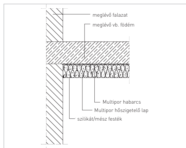
Födém – fal csatlakozás 1.
