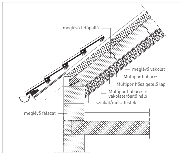
Tetőtér, pallófödém 1.
