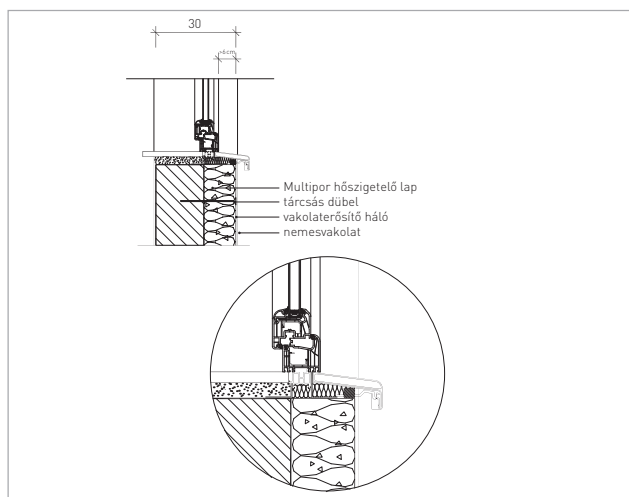
Nyílászáró – függőleges
