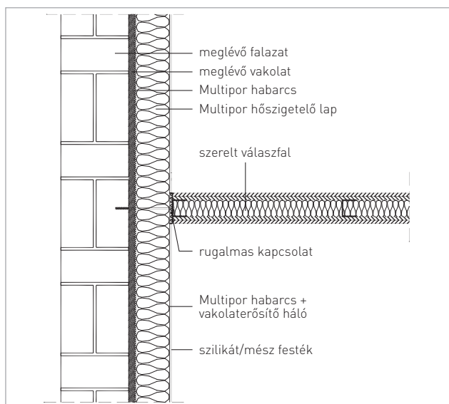
Szerelt válaszfal – vízszintes (b)
