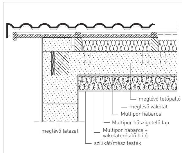
Tetőtér pallófödém 2.
